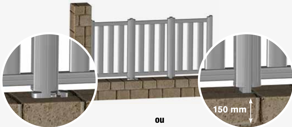
poteau à visser avec platine et cache-boulons intégré
