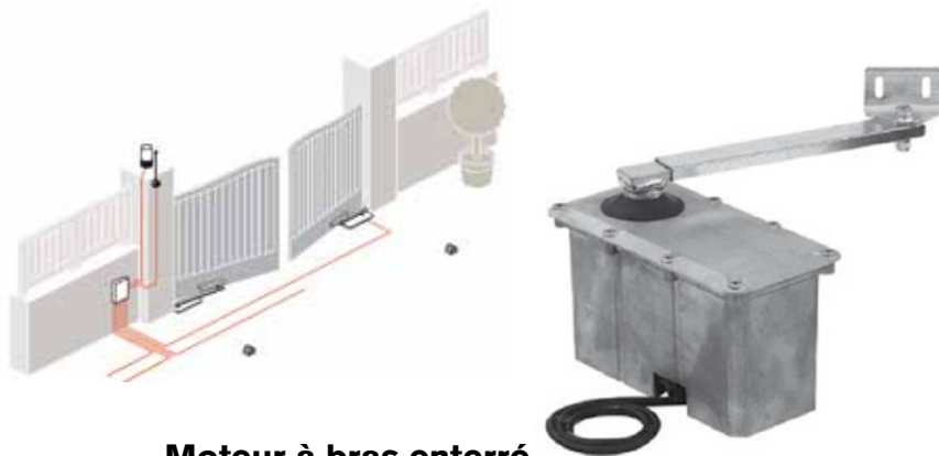
Moteur à bras enterré Renforts soudés en option
