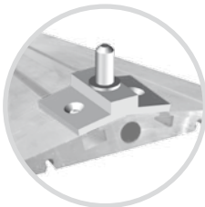
Crapaudine sur seuil aluminium
